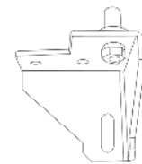
9. Den Stift vom unteren Scharnier abmontieren und das untere Scharnier 90 Grad drehen.
