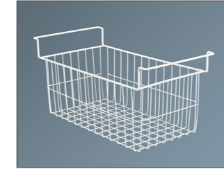
BASKET: KURVC150 (NOT SUITABLE FOR EL 71) W X H: 278 X 196 MM
