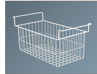
BASKET: KURVC150 (NOT SUITABLE FOR EL 71) W X H: 278 X 196 MM
